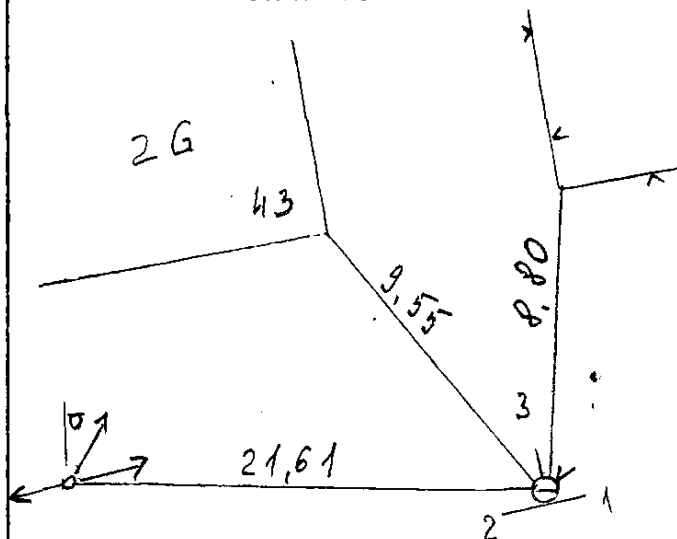
PRIRIŠIMO SCHEMA
