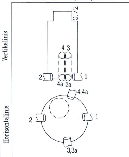
ŠULINIO PJŪVIAI (Matmenys duoti m)
