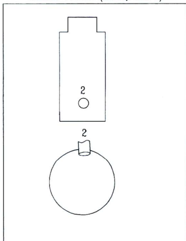
ŠULINIO PJŪVIAI (Matmenys duoti m)
