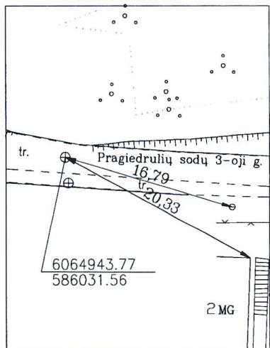
PRIRIŠIMO BRĖŽINYS
