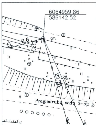
PRIRIŠIMO BRĖŽINYS
