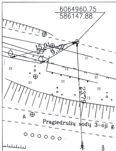
PRIRIŠIMO BRĖŽINYS
