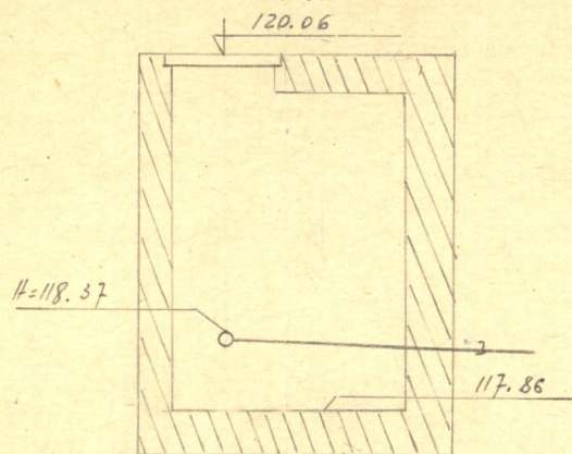
Чертеж колодца М 1:50
