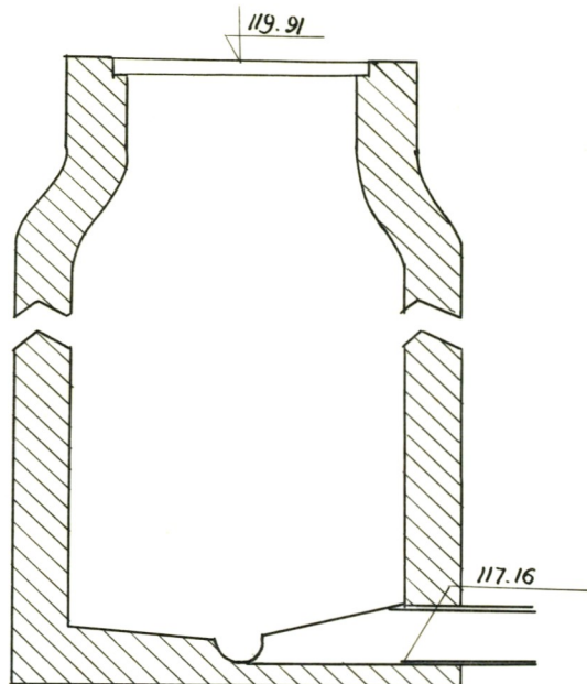
Чертеж колодца М 1:25
