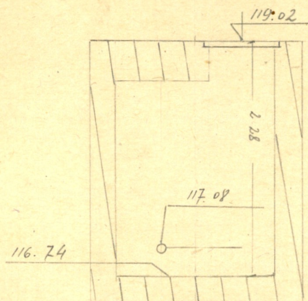
Чертеж колодца М 1:50
