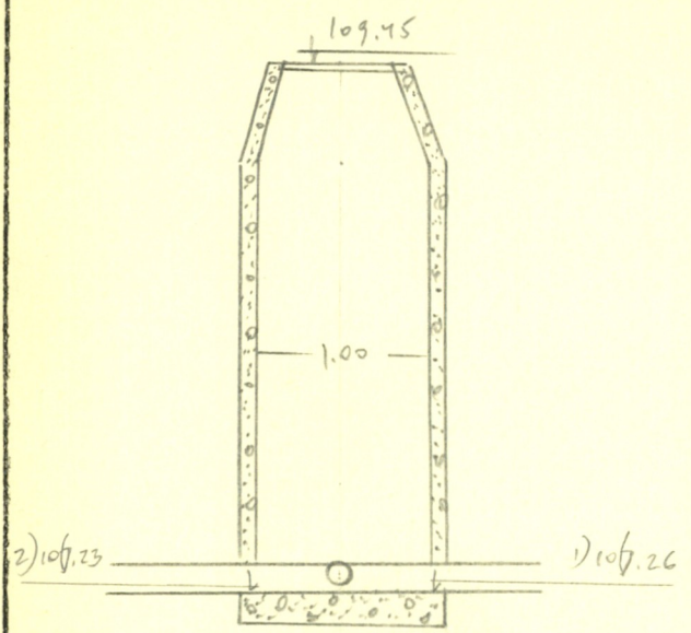
Чертеж колодца М 1: 50
