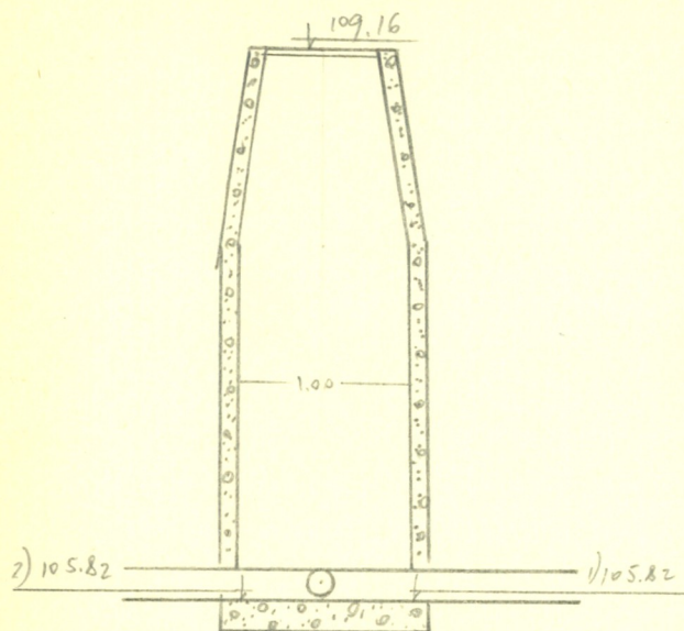
Чертеж колодца М 1:50
