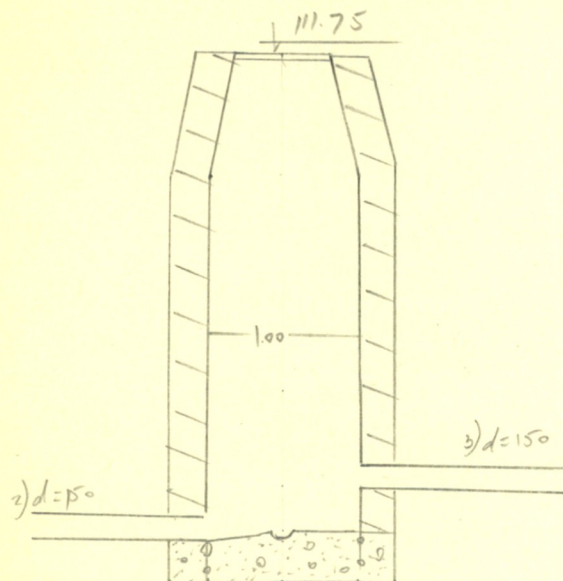
Чертеж колодца М 1: 50
