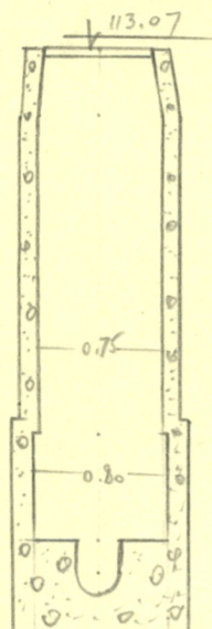
Чертеж колодца М 1:50
