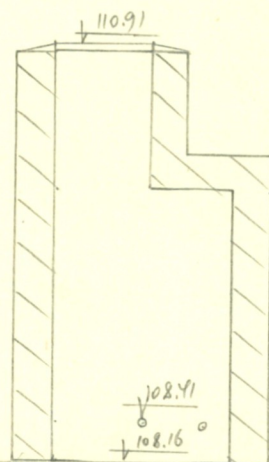
Чертеж колодца М. 1:50
