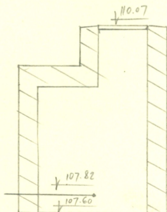
Чертеж колодца М. 1:50
