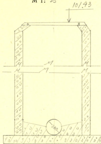
Чертеж колодца М 1: 25
