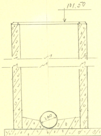
Чертеж колодца М 1:25
