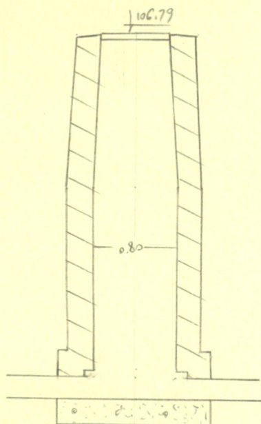
Чертеж колодца М 1:50
