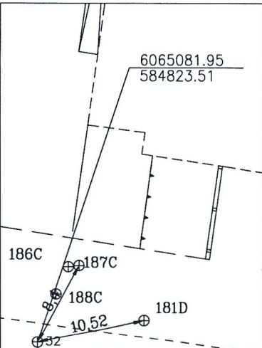
PRIRIŠIMO BRĖŽINYS
