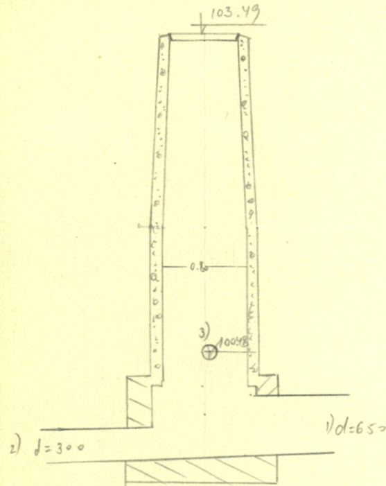
Чертеж колодца М 1:50
