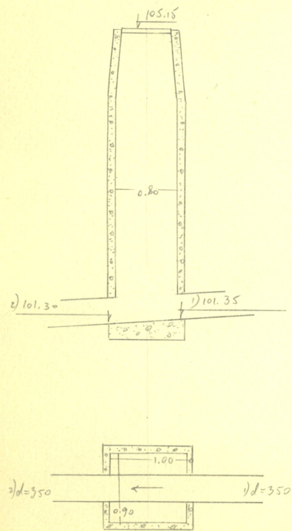
Чертеж колодца М 1:50
