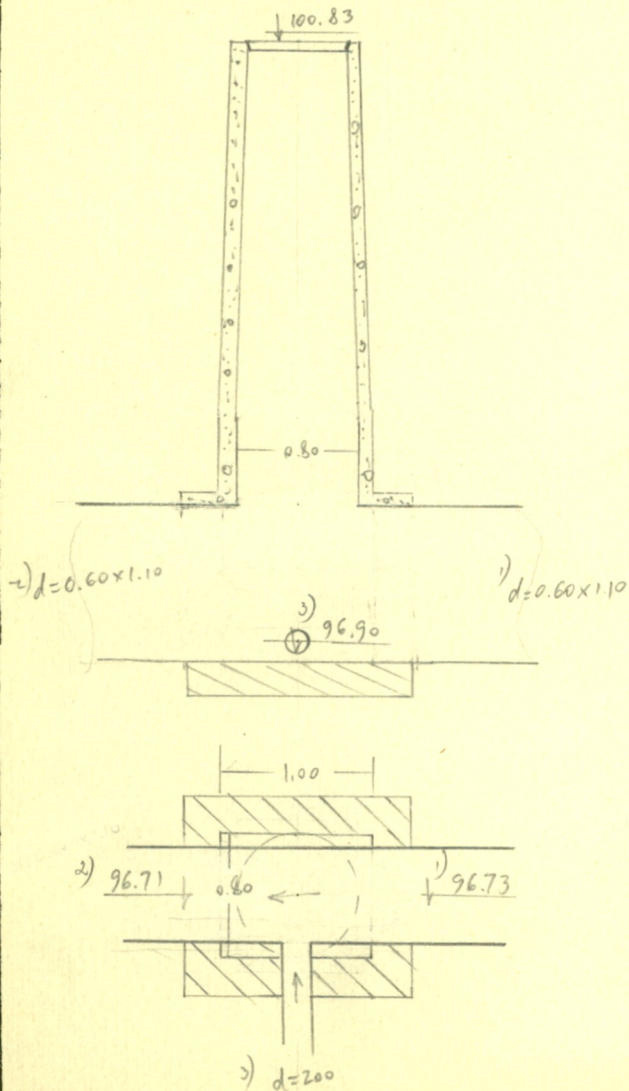
Чертеж колодца М 1:50
