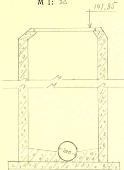
Чертеж колодца М 1: 25
