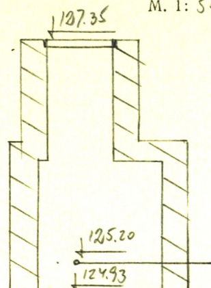
Чертеж колодца М. 1:50
