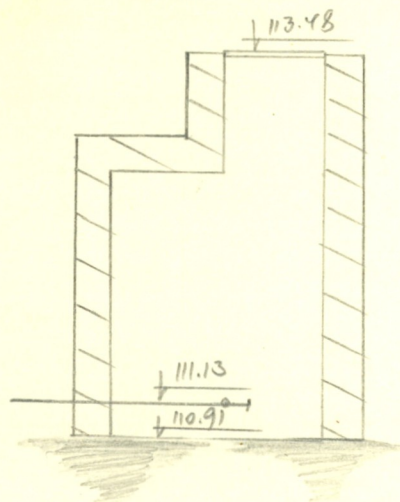
Чертеж колодца М. 1:50
