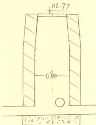
Чертеж колодца М 1:50
