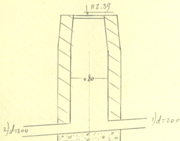
Чертеж колодца М 1:50
