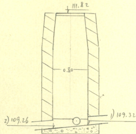
Чертеж колодца М 1: 50
