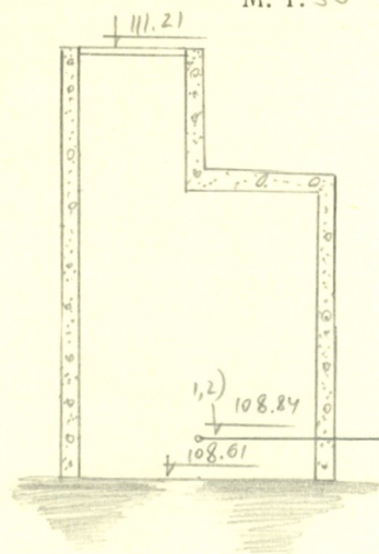
Чертеж колодца М. 1:50
