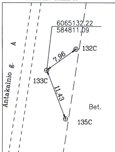
PRIRIŠIMO BRĖŽINYS
