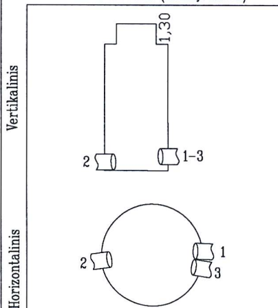
ŠULINIO PJŪVIAI (Matmenys duoti m)
