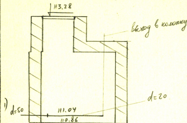
Чертеж колодца М. 1:50
