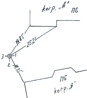
PRIRIŠIMO BRĖŽINYS
