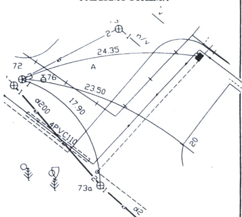
PRIRIŠMO SCHEMA
