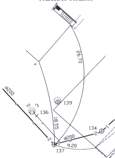
PRIRIŠIMO SCHEMA
