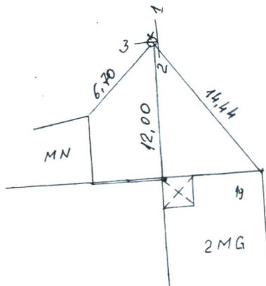
PRIRĖSIMO SCHEMA
