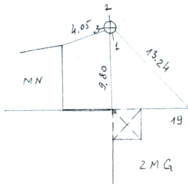
PRIRIŠIMO SCHEMA
