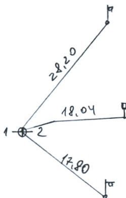
PRIRĖSIMO SCHEMA
