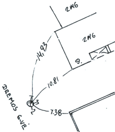
PRIRIŠIMO SCHEMA
