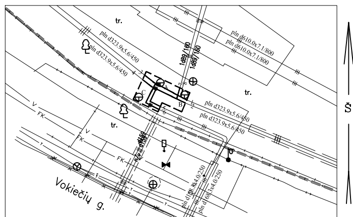
Pririšimo brėžinys
