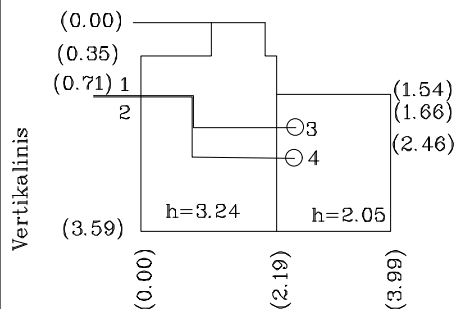
Šulinio pjūviai
