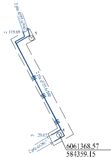
Pririšimo brėžinys
