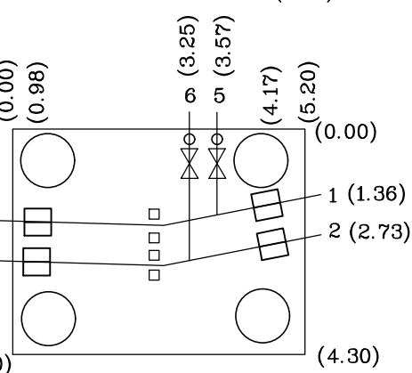
Pririšimo brėžinys
