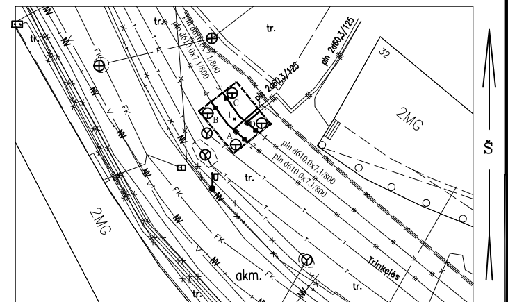
Pririšimo brėžinys
