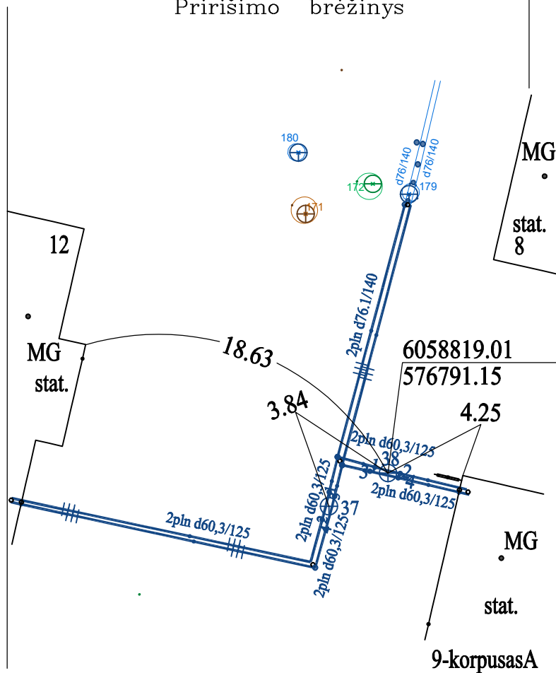
Pririšimo brėžinys
