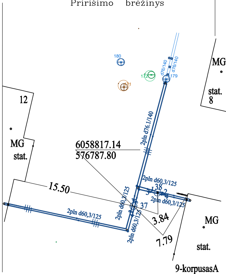
Pririšimo brėžinys
