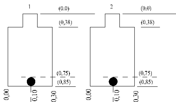
Šulinio pjūviai
