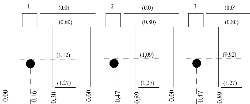
Šulinio pjūviai
