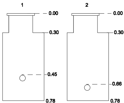
Šulinio pjūviai :
