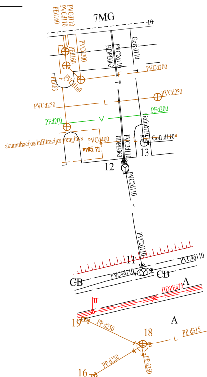
Pririšimo brėžinys:
