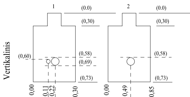
Šulinio pjūviai :
