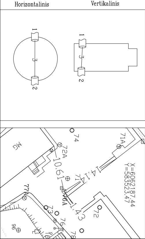
ŠULINIO PLOVIAI (Matmenys duoti m) PRIRIŠIMO BRĖŽINYS
