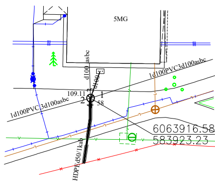
Pririšimo brėžinys
