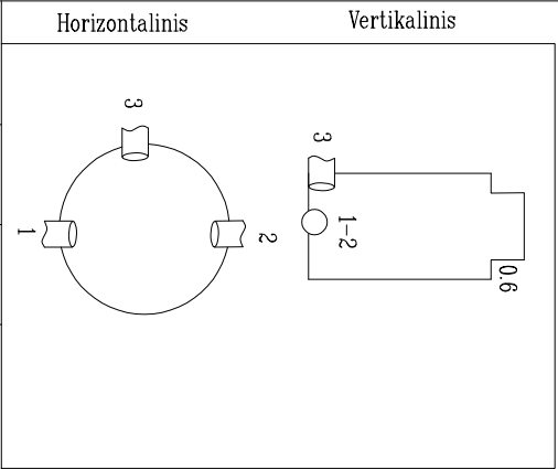
ŠULINIO PIJŲVAI (Matmenys duoti m)
